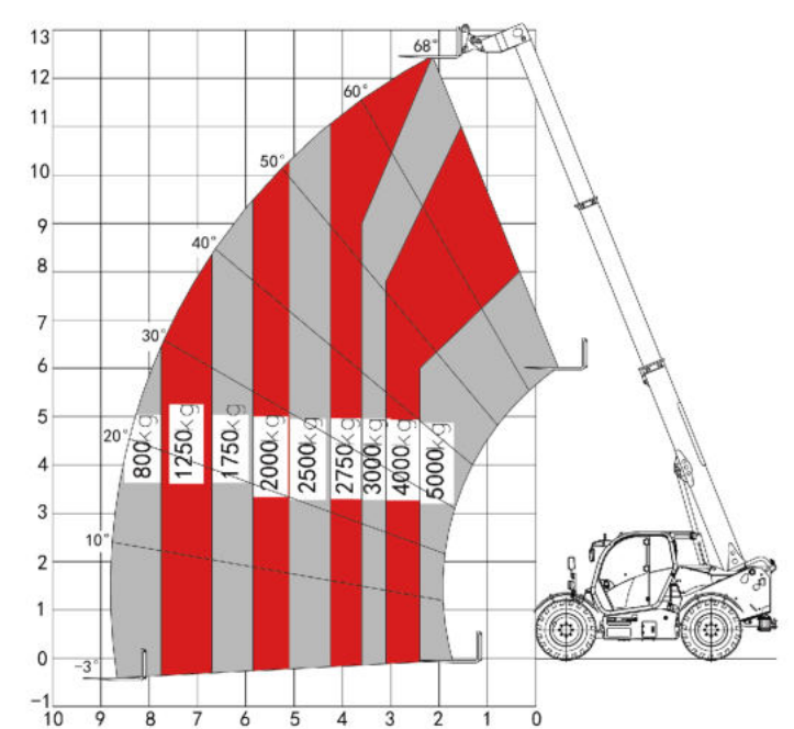
50THCJ13-Q/Q1/CU 载荷曲线图 Lifting diagram
