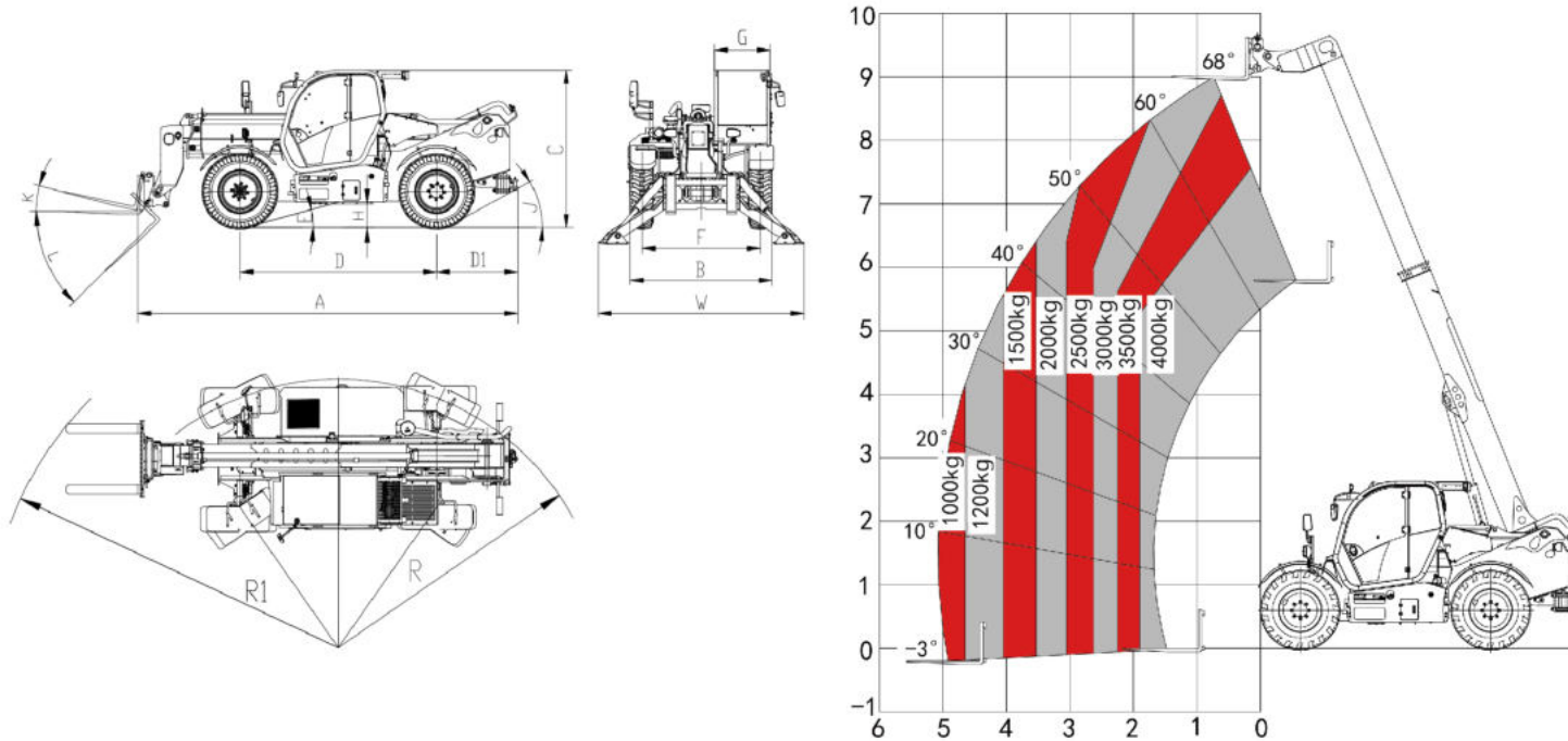
40THCJ09-Q/Q1/CU 尺寸参数 Dimension
