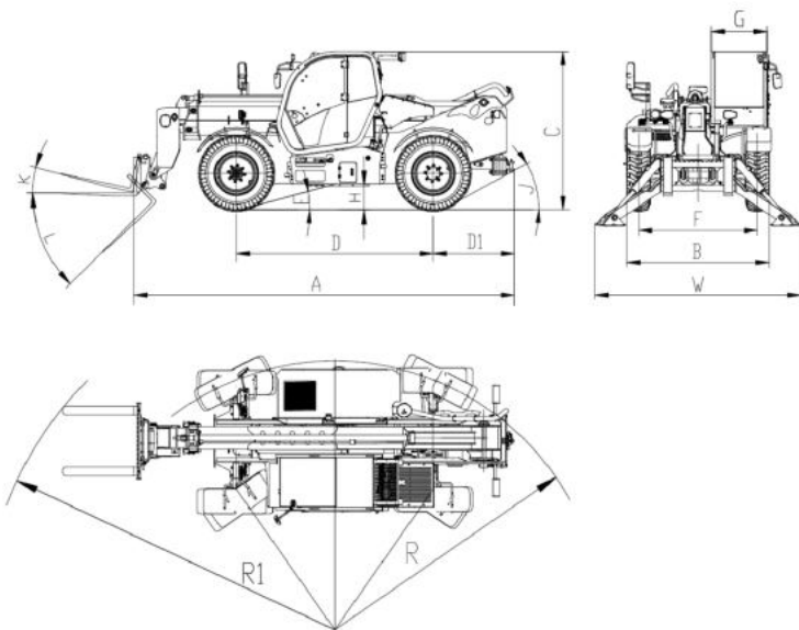
35THCJ09-Q/Q1/CU 尺寸参数 Dimension
