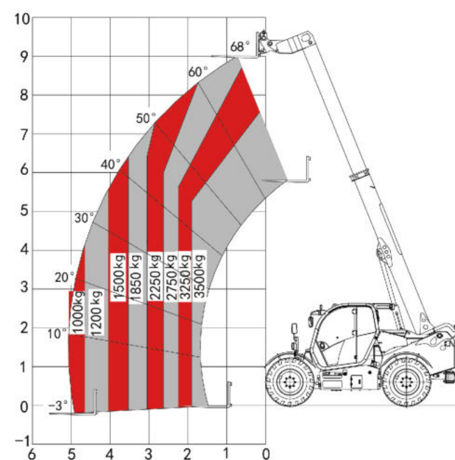
35THCJ09-Q/Q1/CU 载荷曲线图 Lifting diagram
