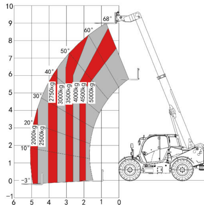
50THCJ09-Q/Q1/CU 载荷曲线图 Lifting diagram
