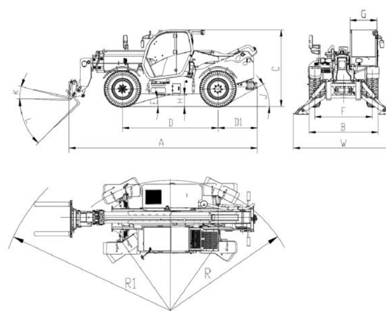
35THCJ13-Q/Q1/CU 尺寸参数 Dimension
