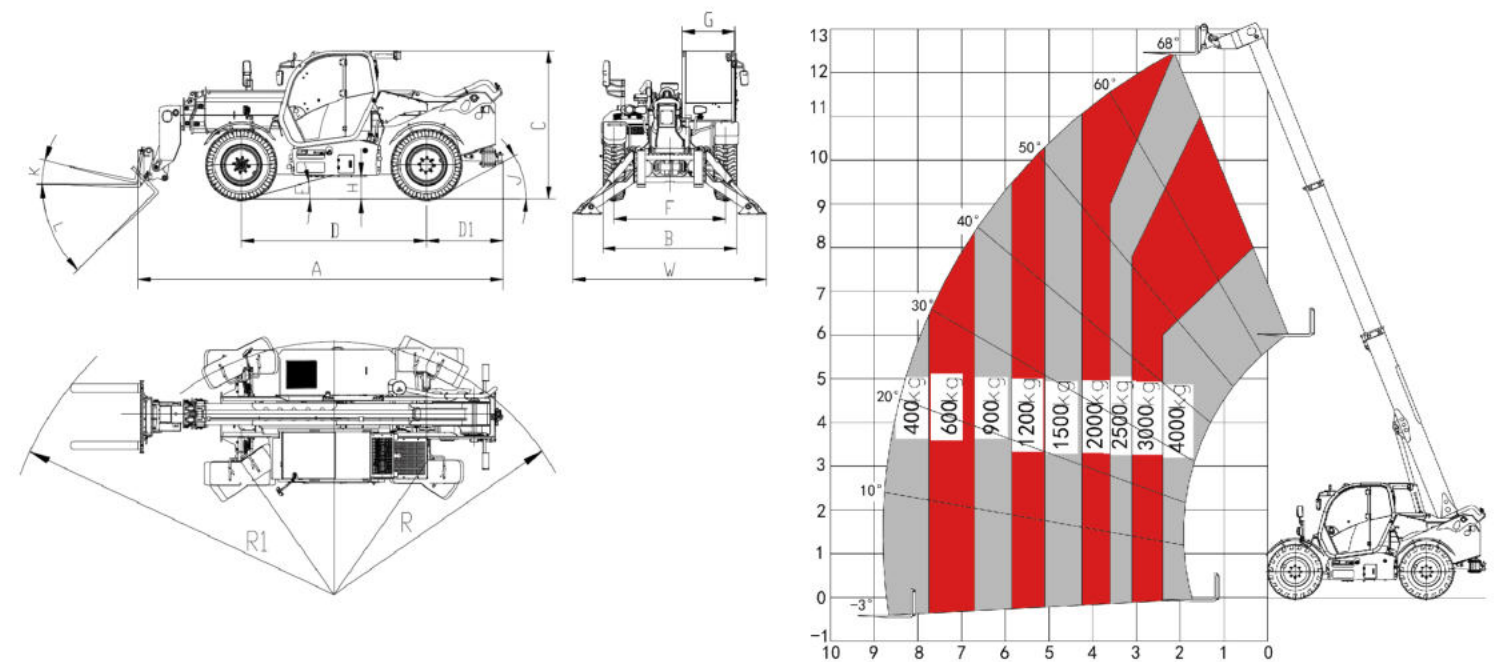
40THCJ13-Q/Q1/CU 尺寸参数 Dimension
